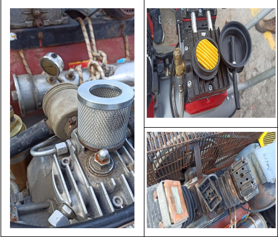
Şekil 2: Şekil Hava emiş filtre tipleri
