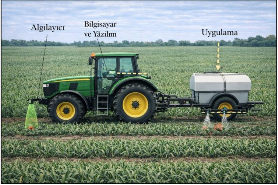
Şekil 2. Algılayıcı esaslı sistemin çalışma prensibi
