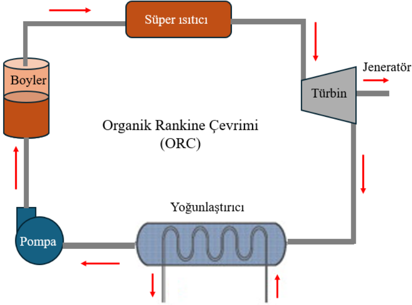
Şekil 4. Organik Rankine Çevrimi (ORC) [9]
