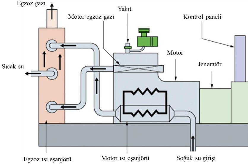
Şekil 5. Gaz motorlu CHP sistemi
