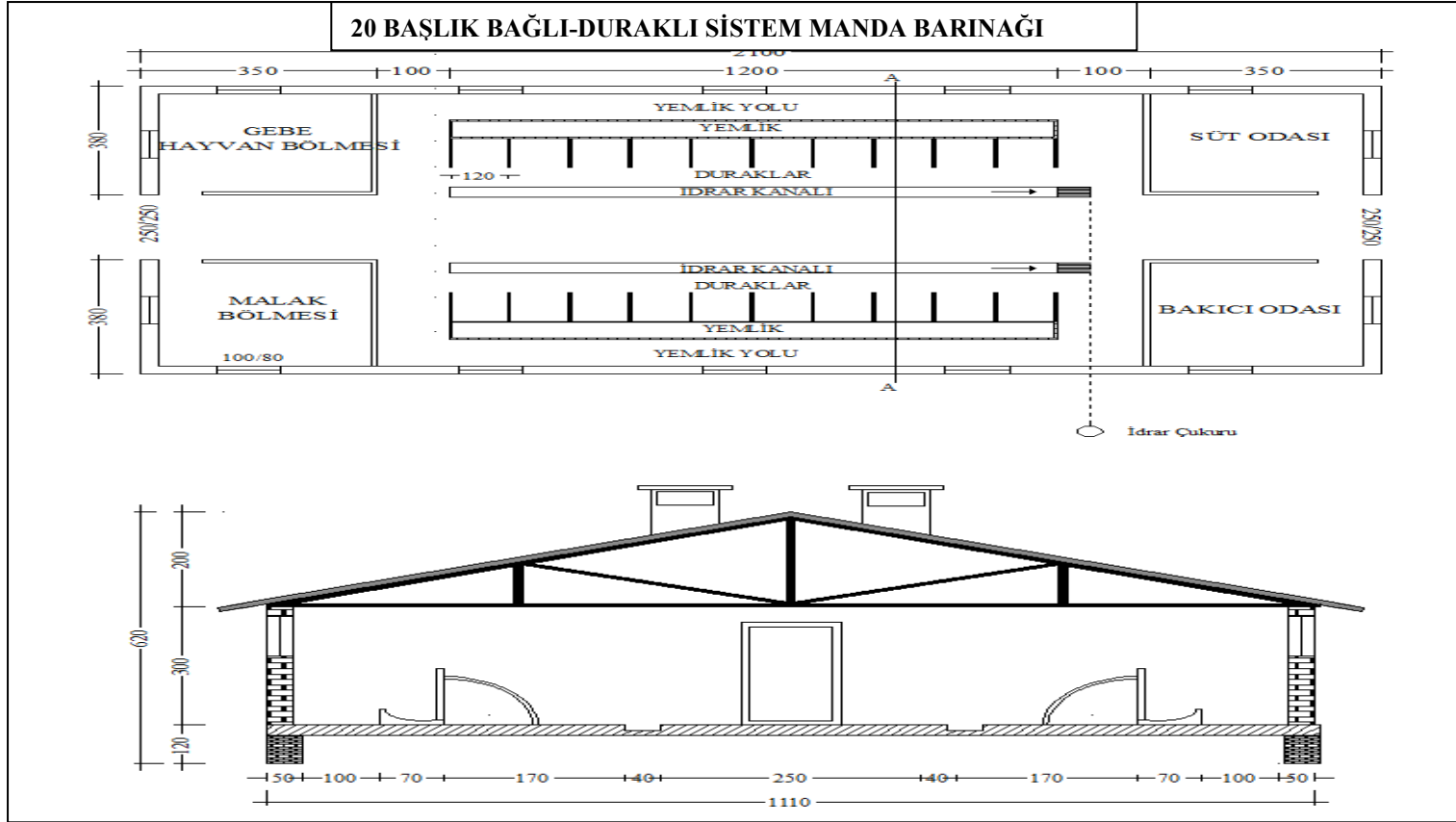
Şekil 11. Yirmi başlık bağlı-duraklı sistem manda barınağı taban planı ve kesit görünüşü
