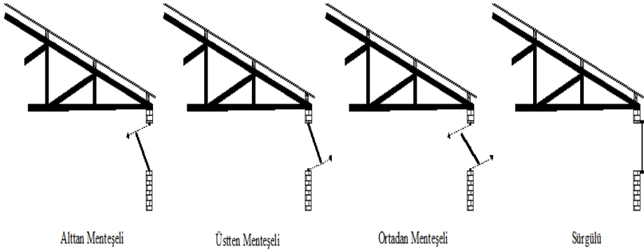
Şekil 4. Hayvan barınaklarında uygulanan havalandırma panelleri
