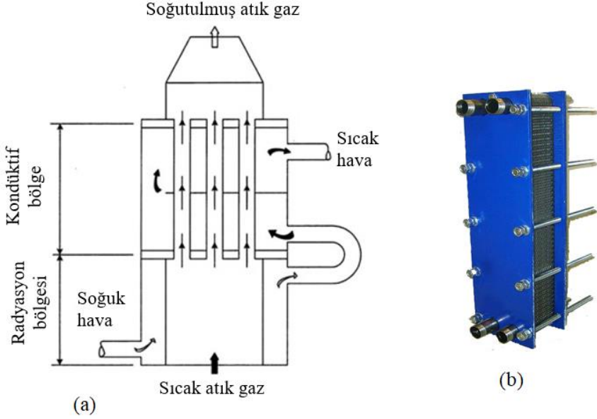
Şekil 1. Borulu reküperatör sisteminin çalışma prensibi (a) ve plakalı reküperatör (b) [2]
