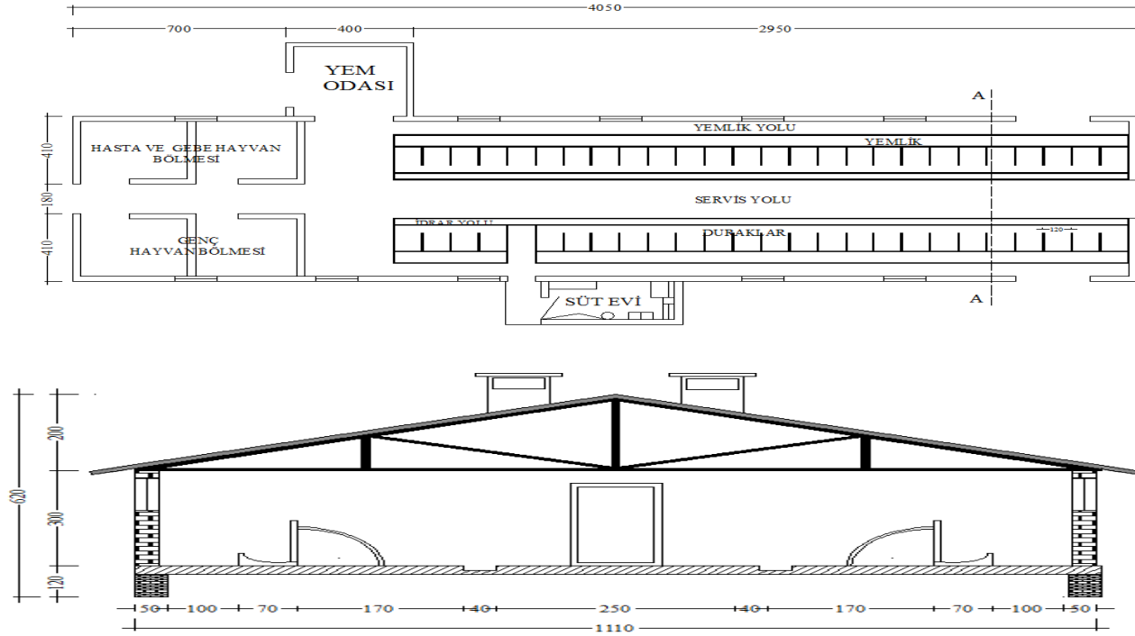
Şekil 12. Elli başlık bağlı-duraklı sistem manda barınağı taban planı ve kesit görünüş
