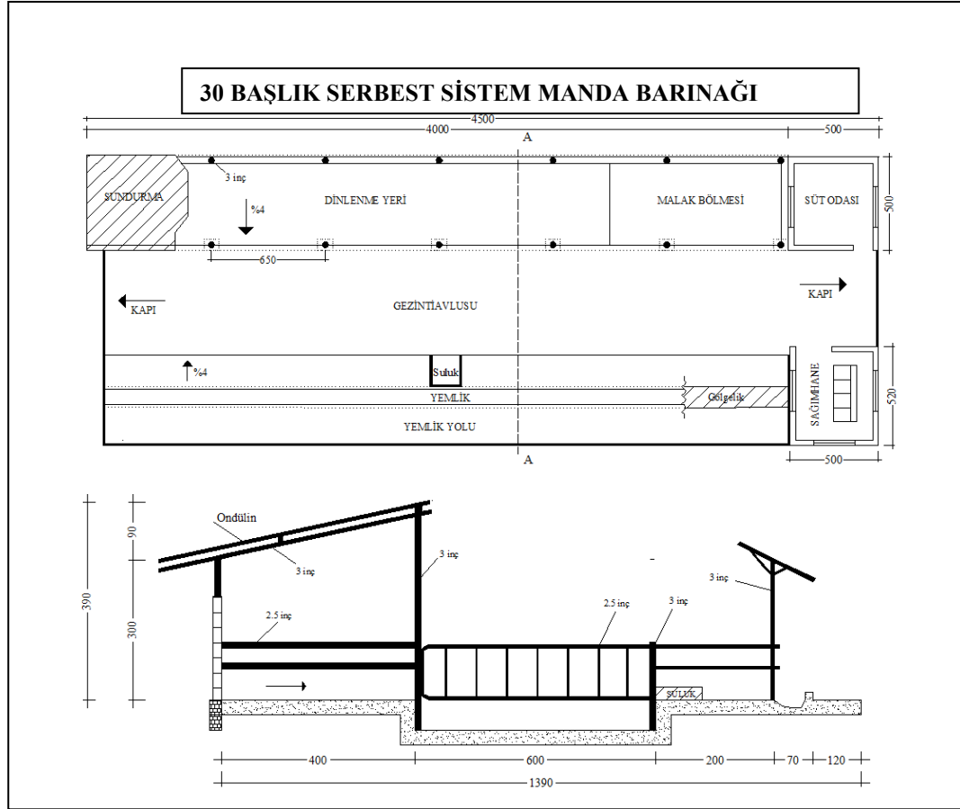
Şekil 9. Otuz başlık serbest sistem manda barınağı taban planı ve kesit görünüşü
