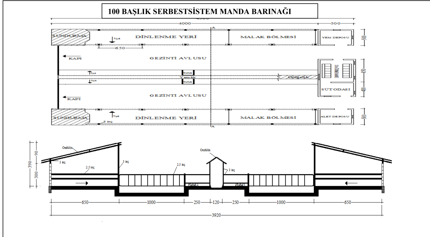
Şekil 10. Yüz başlık serbest sistem manda barınağı taban planı ve kesit görünüşü
