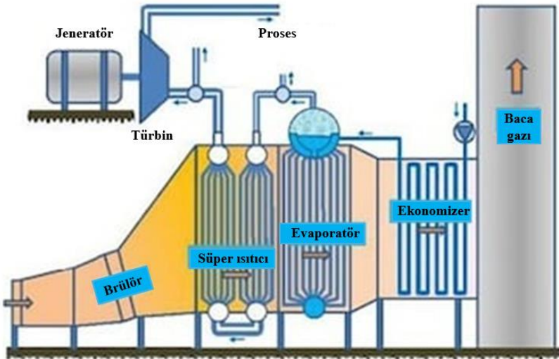
Şekil 3. Buhar kazanlarında borulu tip ekonomizer kullanımı
