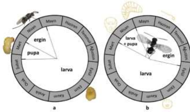
Şekil 2. Torymus sinensis (a) ve konukçusu olan Dryocosmus kuriphilus 'un yaşam döngüsü (b) (İpekdağ ve ark., 2017).
