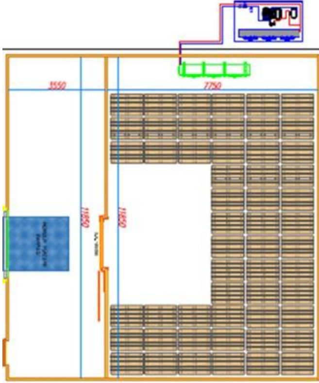
Şekil 1. Soğuk deponun genel görünümü ve boyutları
