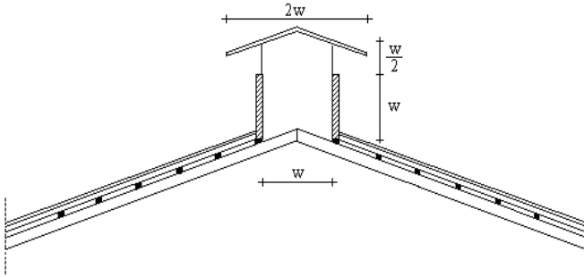
Şekil 7. Fener tipi hava çıkış açıklığı kesit görünüşü
