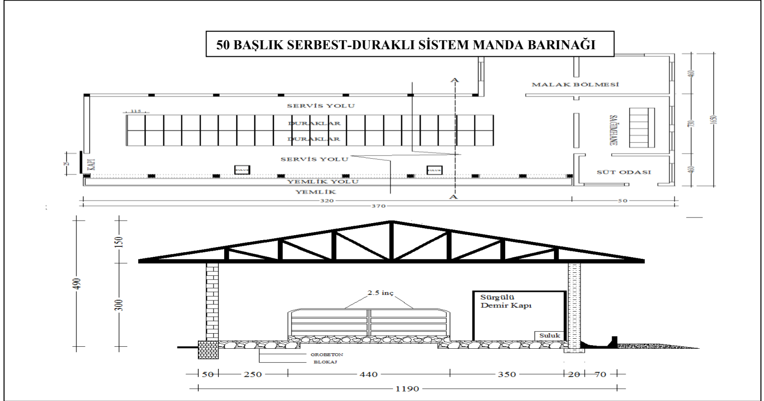
Şekil 13. Elli başlık serbest-duraklı sistem manda barınağı taban planı ve kesit görünüşü
