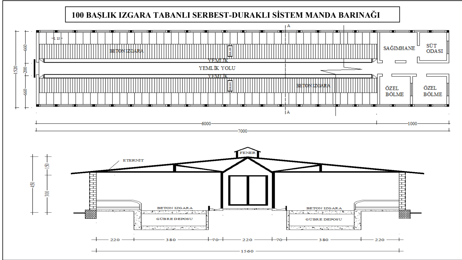
Şekil 14. Yüz başlık ızgara tabanlı serbest-duraklı sistem manda barınağı taban planı ve kesit görünüşü
