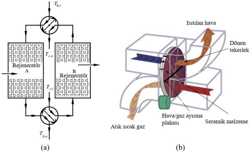
Şekil 2. Sabit yataklı (a) ve döner (b) rejeneratörler [4], [5]
