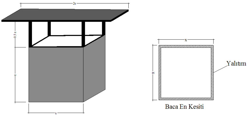
Şekil 5. Havalandırma bacasının perspektif görünüşü
