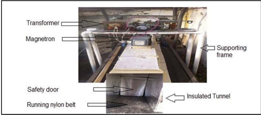
Şekil 4: Rana ve Derr (2017)'in çalışmasında kullanılan düzenek
