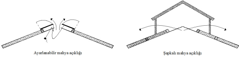
Şekil 6. Mahya açıklığı tipleri
