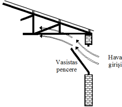
Şekil 1. Hava giriş açıklığı olarak kullanılan vasistaslı pencere
