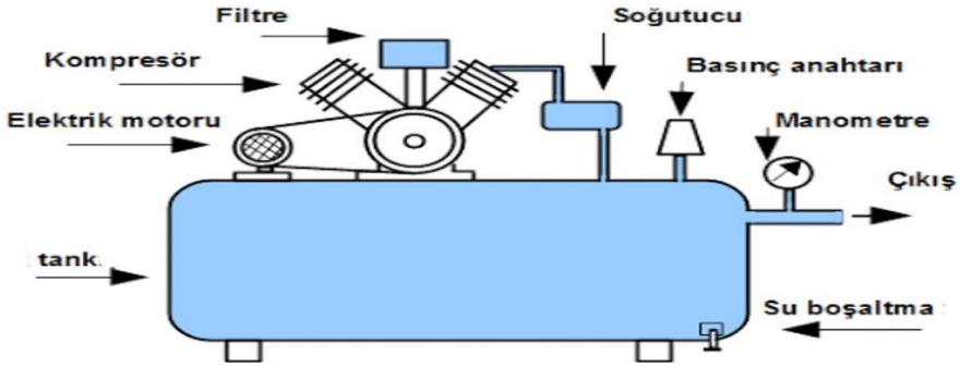
Şekil 1: Alçak basınç kompresörünün genel yapısı
