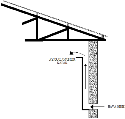
Şekil 3. Barınaklarda farklı tipteki hava giriş deliklerinin kullanımı
